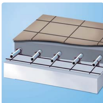
Система с арматурной сеткой Uponor Classic
