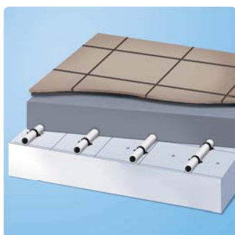
Система креплений степлером Uponor Tacker
