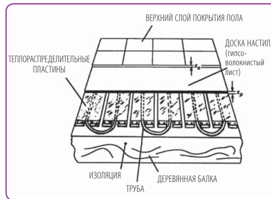
Рисунок 3.11 Теплораспределительная пластина для деревянных полов
